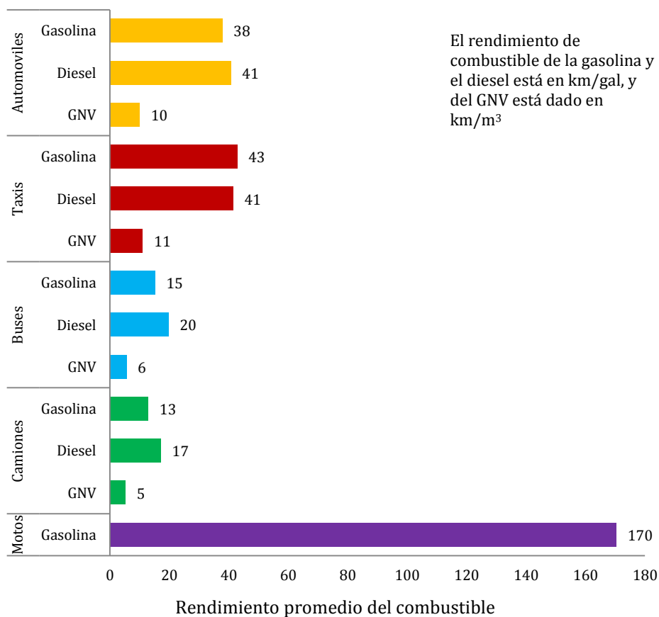
Figura 3.6. Rendimiento promedio ponderado del combustible, año 2011
