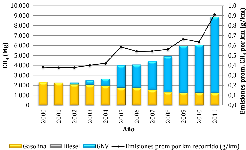
Figura 3.35. Evolución de las emisiones de metano (CH 4 )
