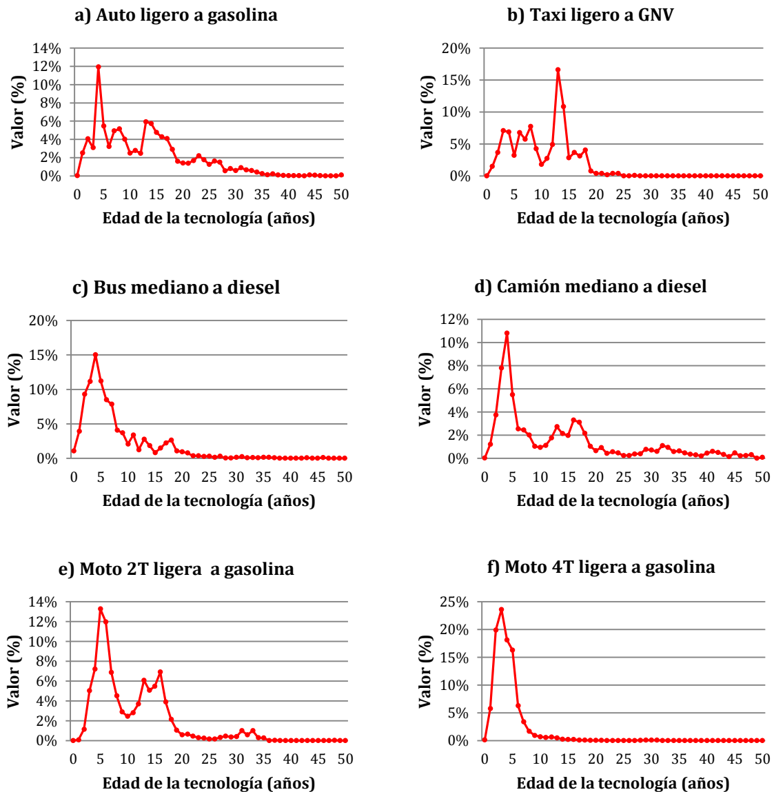
Figura 3.2. Perfiles de antigüedad de algunas tecnologías
