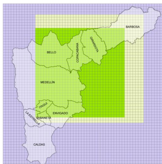
Figura 2.1. Dominios del modelo MODEAM
